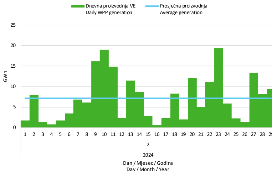
Slika 5 Dnevna proizvodnja svih vjetroelektrana u veljači 2024. godine Figure 5 Daily generation of all wind power plants in February 2024
