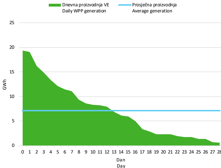
Slika 6 Krivulja trajanja dnevne proizvodnje vjetroelektrana u veljači 2024. godine Figure 6 Average daily WPP generation duration curve in February 2024
